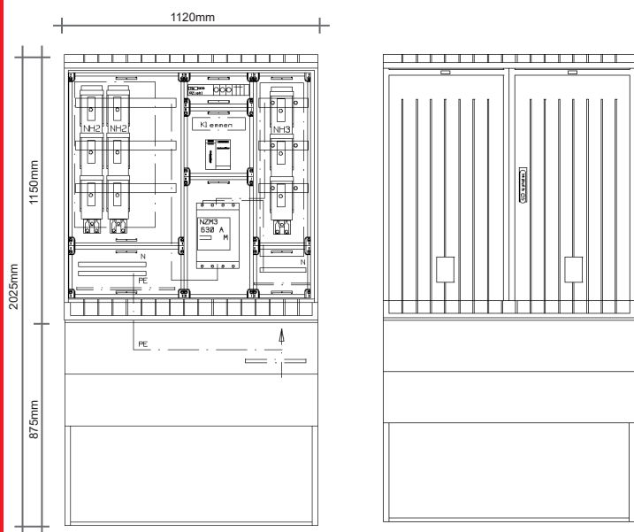
BxHxT = 1120mm x 1150mm x 320mm (Gehäuse ohne Sockel)
