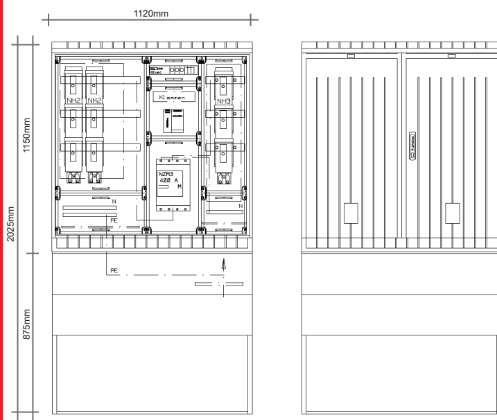
BxHxT = 1120mm x 1150mm x 320mm (Gehäuse ohne Sockel)
