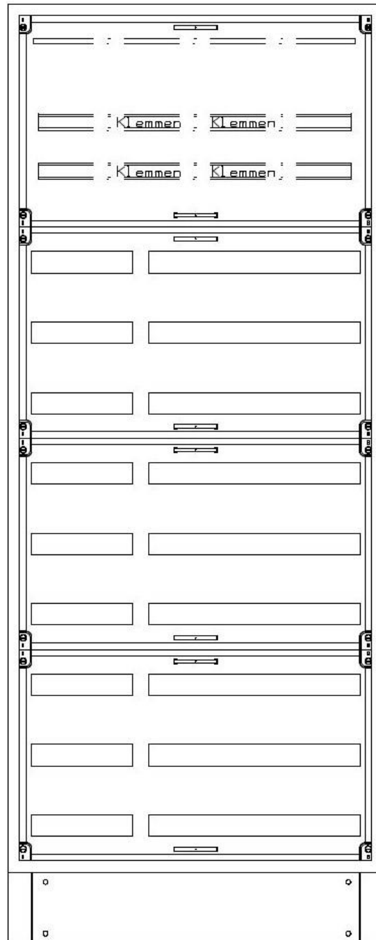
Bild einer Standverteilung SVK3-12-300 mit Standard-Geräteträger und Feldabdeckungen PRL
